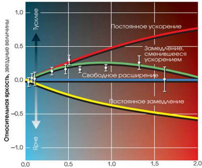
Рис. 1. Красное смещение.
